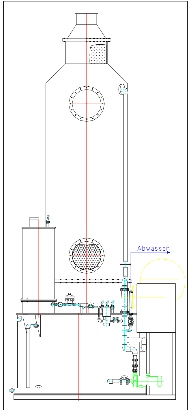
Vertikalabgaswäscher
