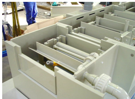
Abbildungen: Versuchsträger zum Testen eines neuen Verfahrens zur Horizontalabscheidung von Bleiband
